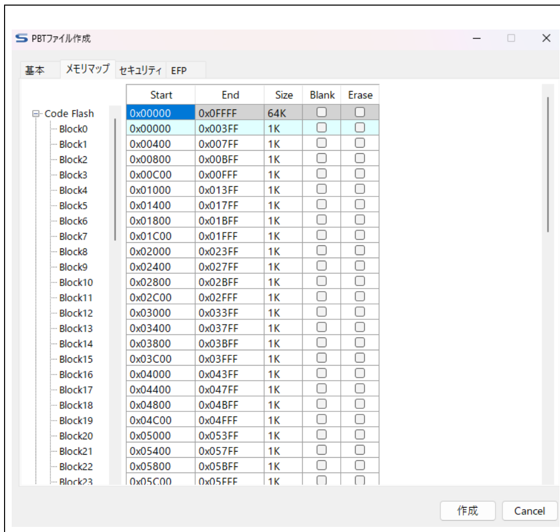
図 2.2 メモリマップタブ
