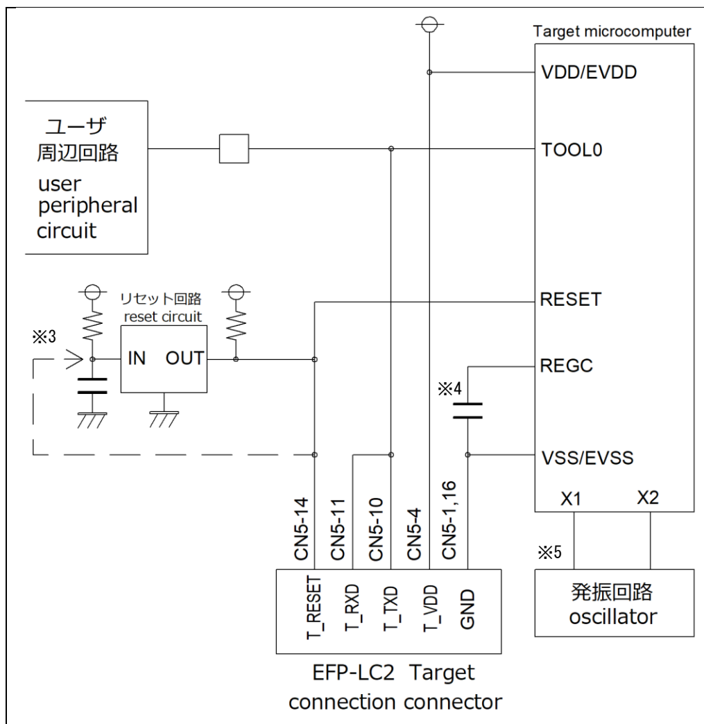
図 1.2 ターゲットシステム推奨回路図
