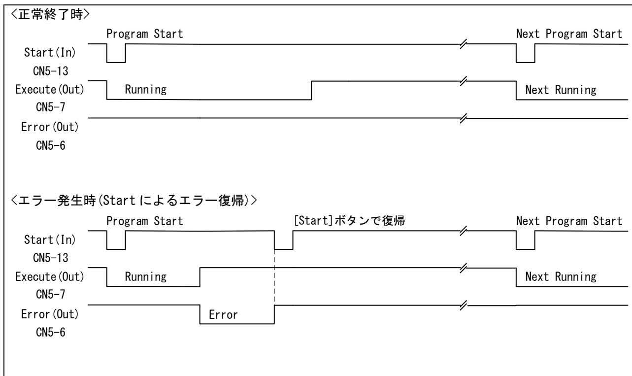
図 1.6 外部制御信号シーケンス
