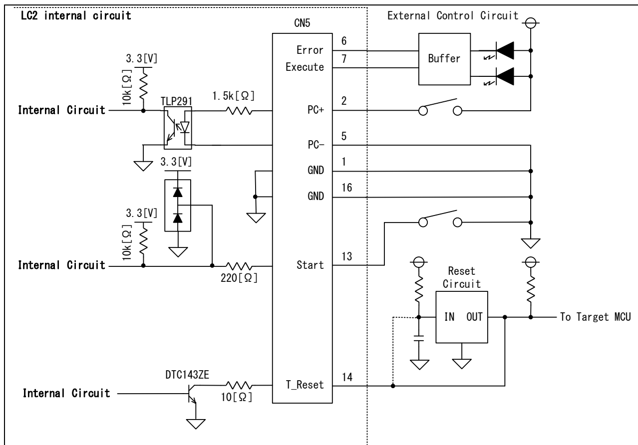
図 1.5 外部制御信号接続例
