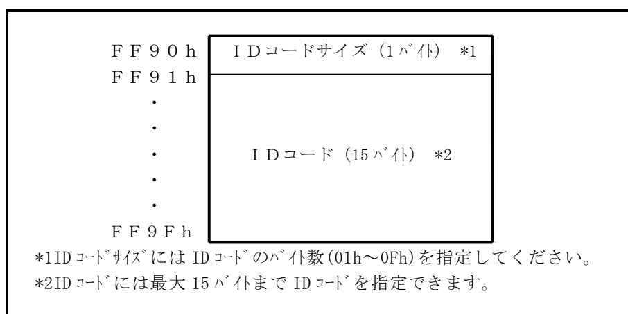
図 5. 1 IDコード領域の構成
