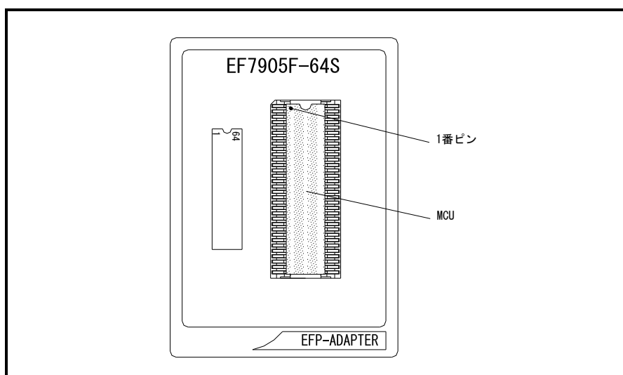
図 2.1 MCUの挿入方向
