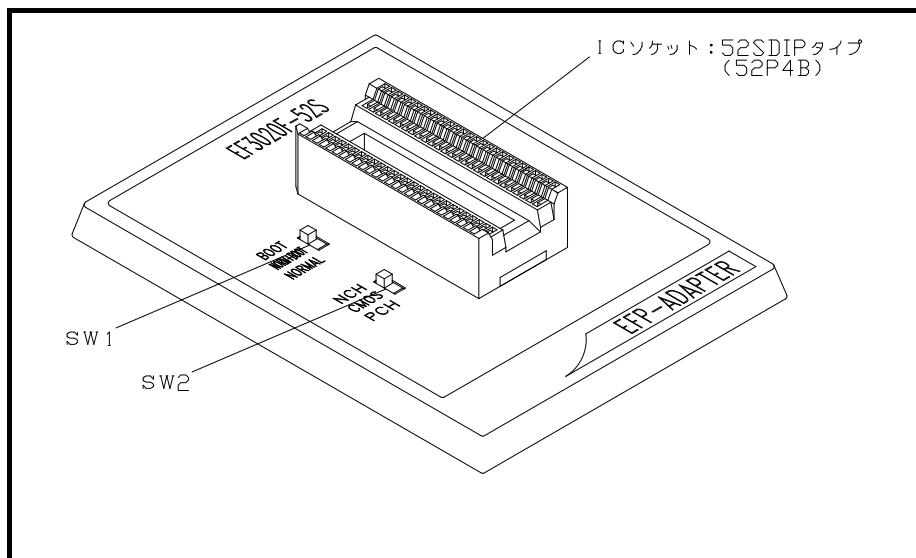
図1.1 EF3020F-52S外形図
