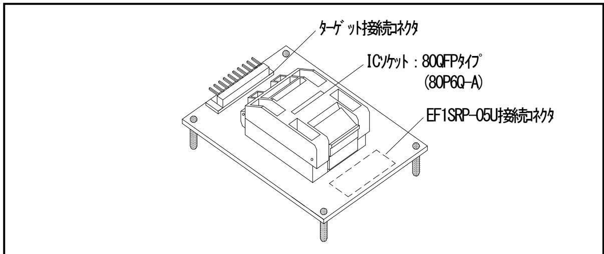
図1. 1 MS3882-80H外形図
