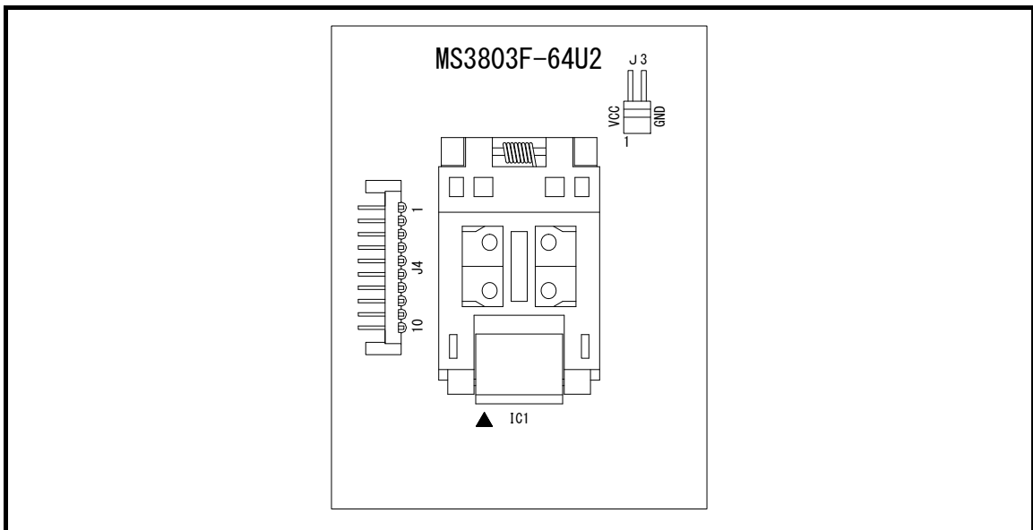
図1. 1 MS3803F-64U2外形図
