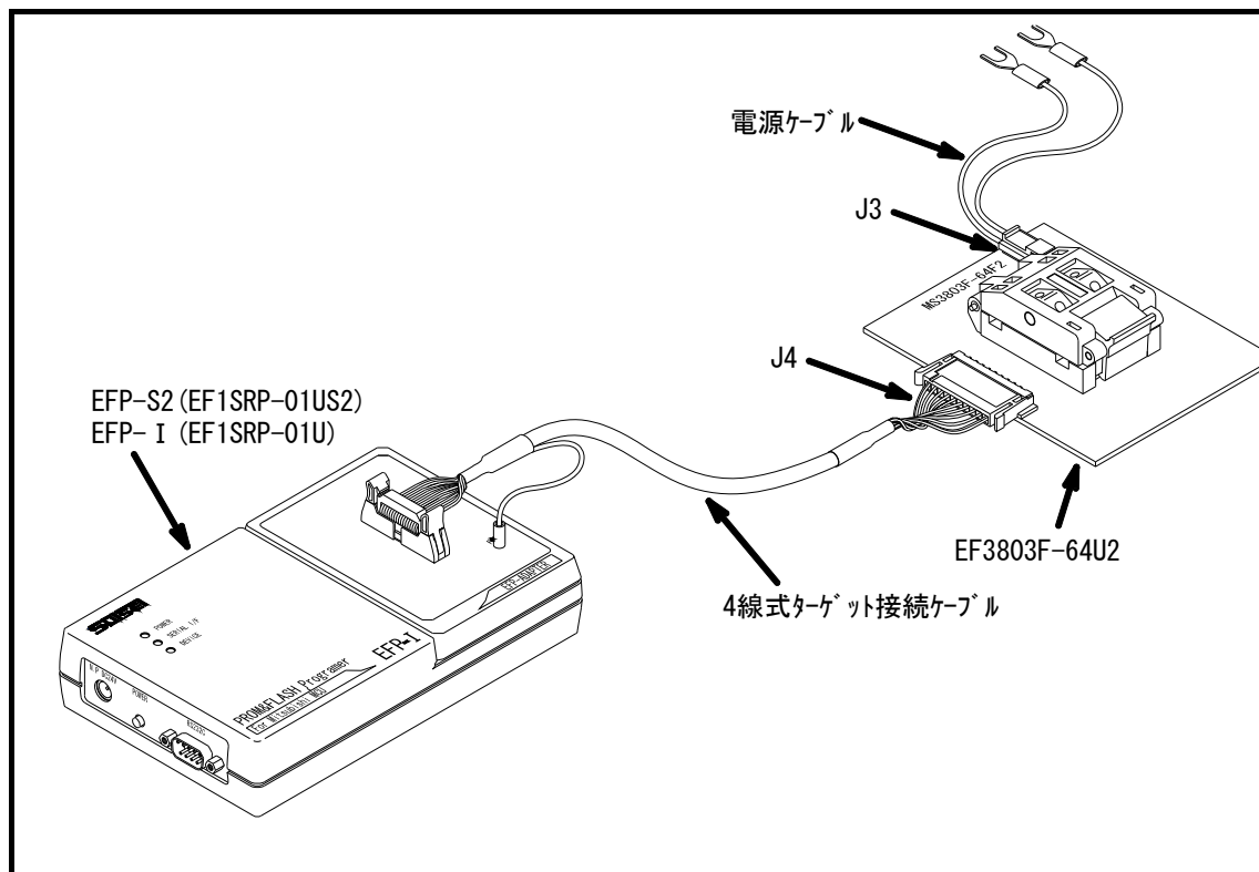
図4. 1 MS3803F-64U2との接続
