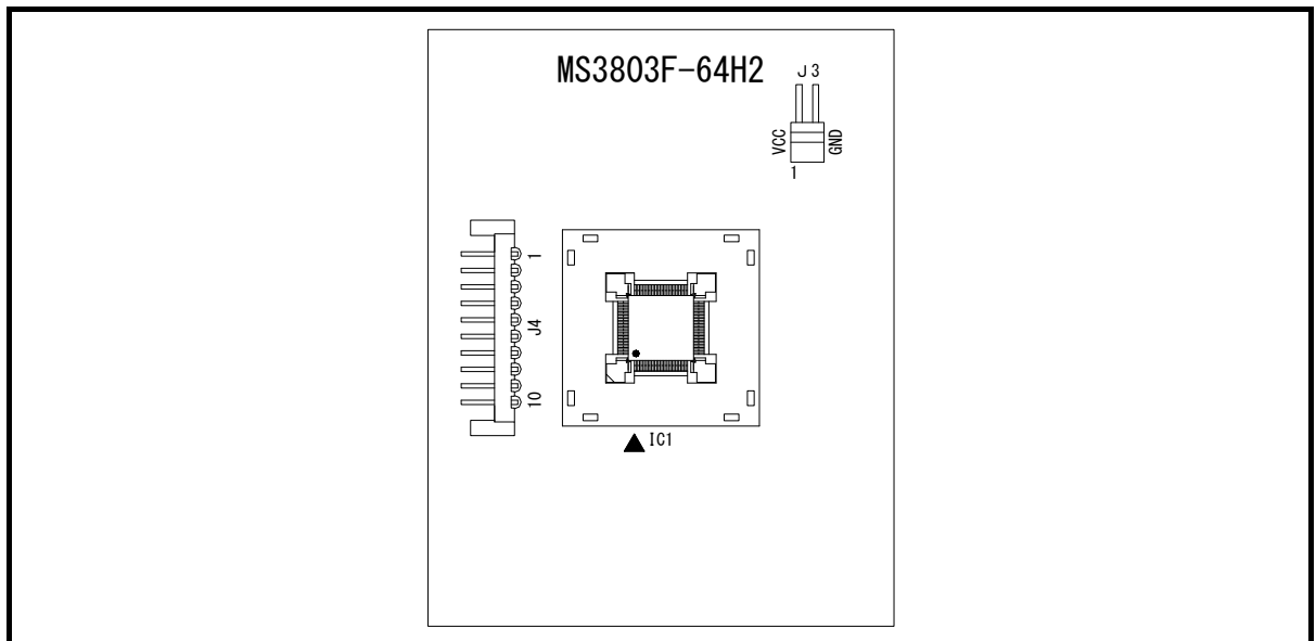
図1. 1 MS3803F-64H2外形図
