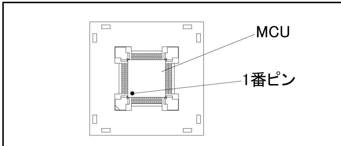
図2. 1 MCUの挿入方法
