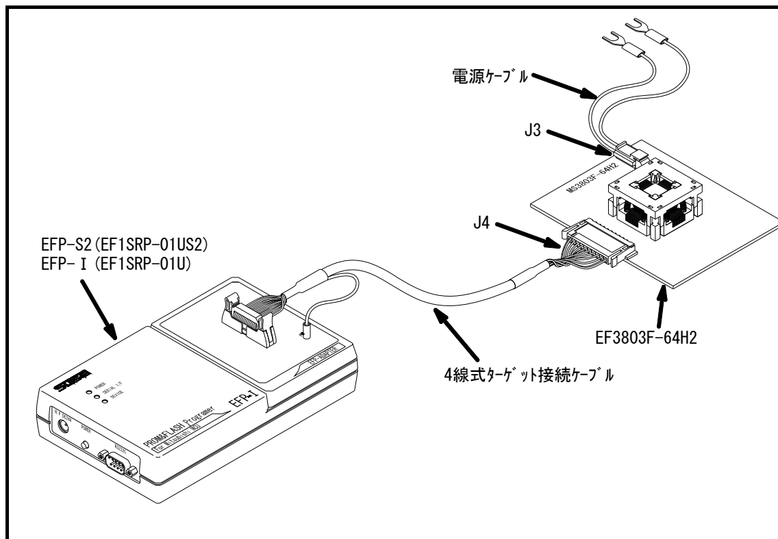
図4. 1 MS3803F-64H2との接続
