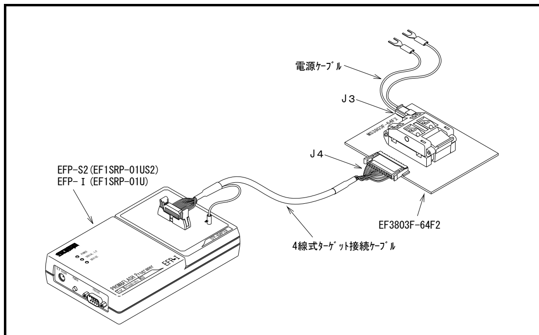
図4. 1 MS3803F-64F2との接続
