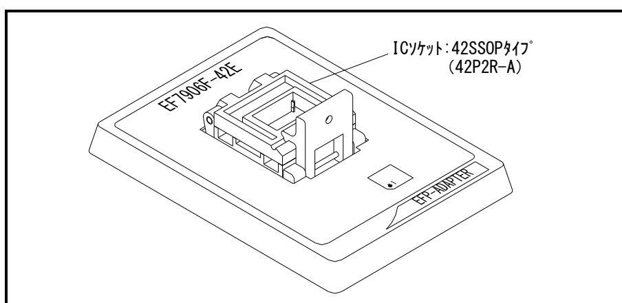
図 1.1 EF7906F-42E 外形図
