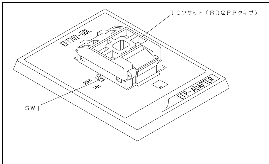
図1.1 EF7702-80L外形図
