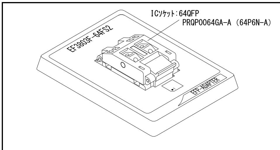
図1. 1 EF3803F-64FS2外形図
