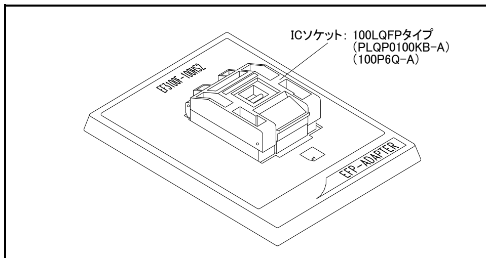
図 1.1 EF3100F-100HS2 外観図
