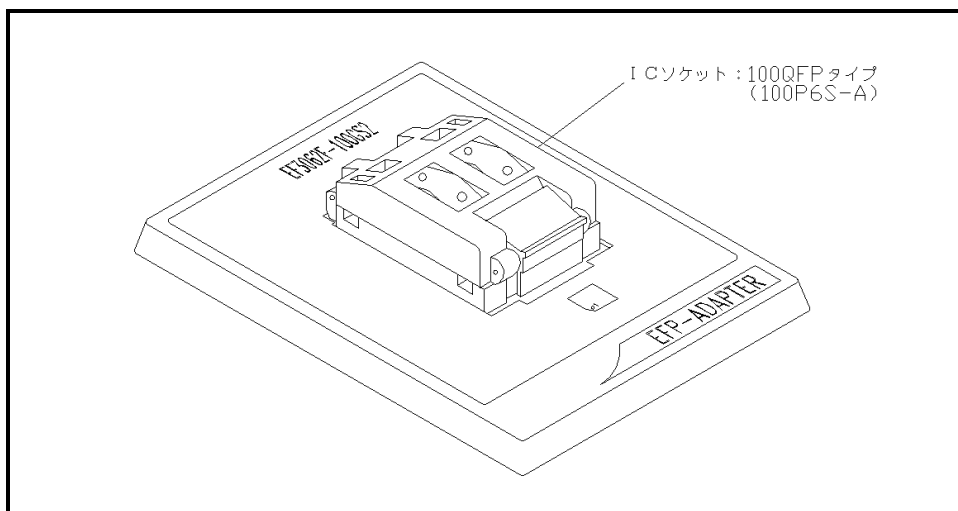
図1. 1 EF3062F-100GS2外形図
