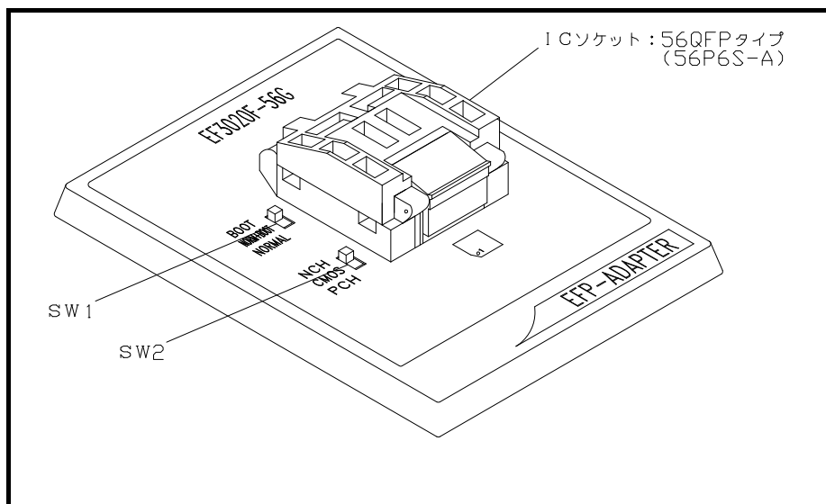
図1. 1 EF3020F-56G外形図
