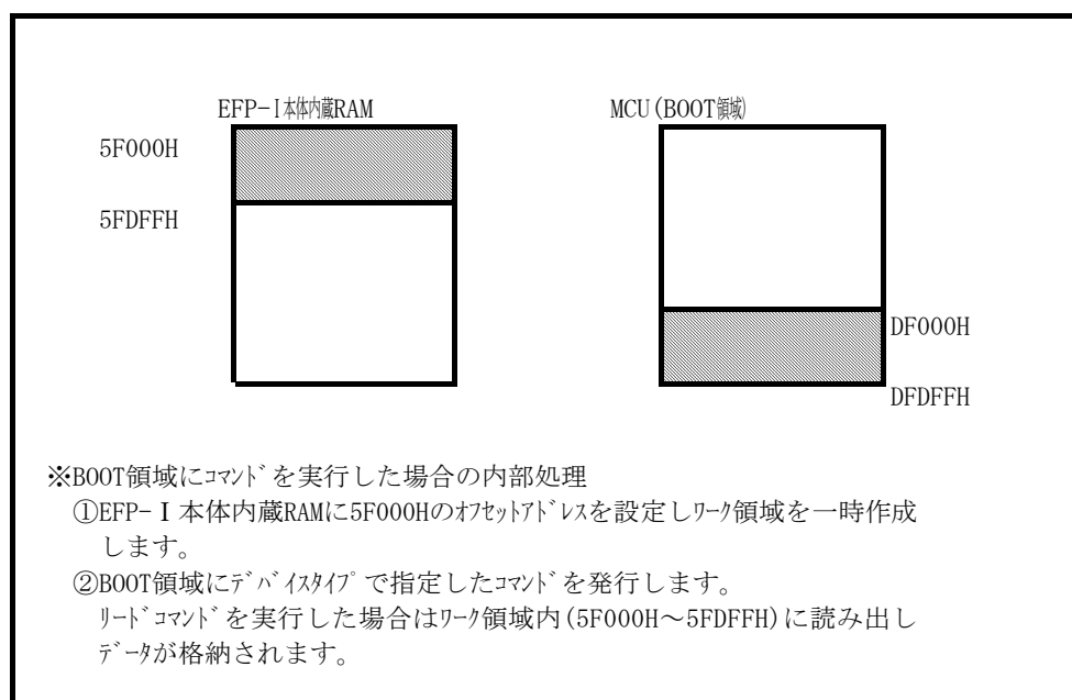
図6.2 ワーク領域概略図
