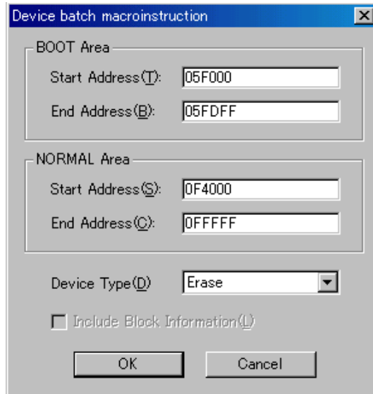
図6.1 デバイス一括マクロコマンドパラメータ入力ダイアログ
